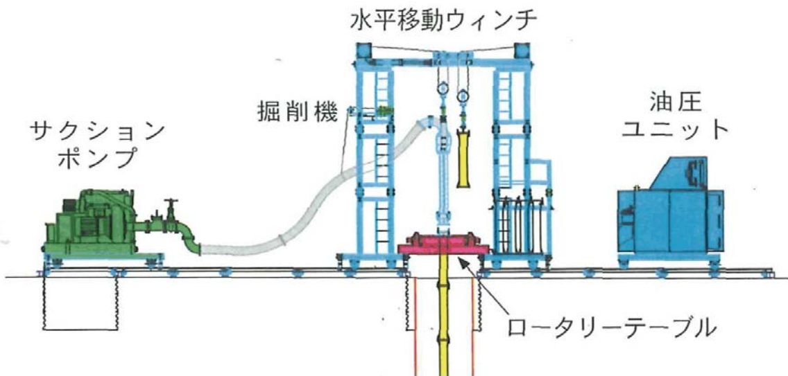
TYPE 2 ロータリーテーブル機構
